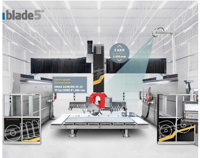
Fresadora até Z 1.600 mm ø 1.200
