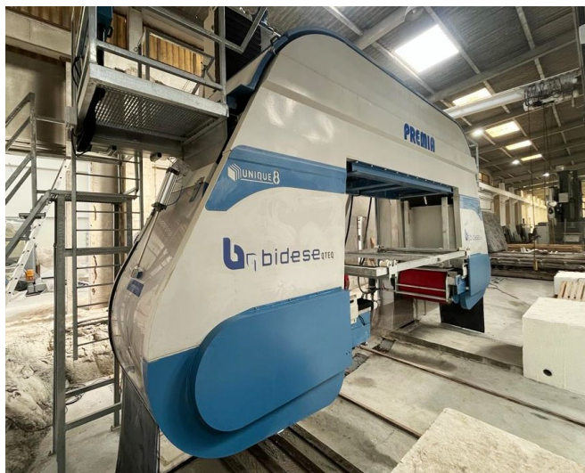
MULTIFIOS com fios de diâmetro 4,3 - 5,3 - 6,3 - 7,3
