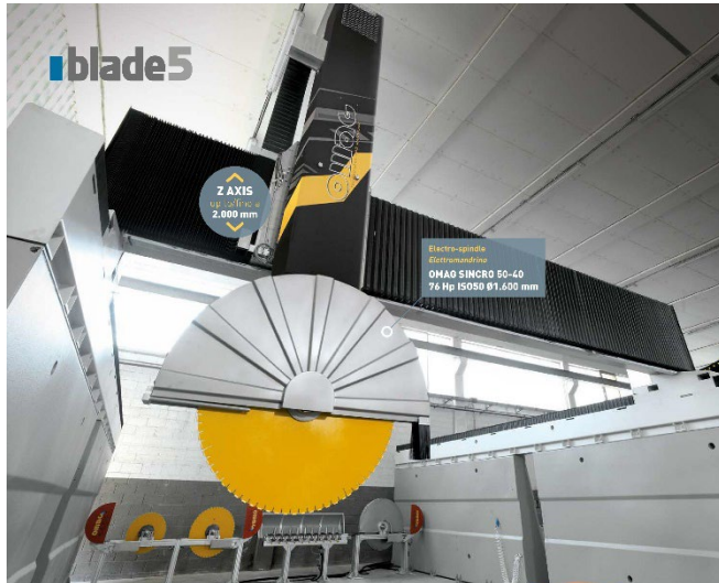
Fresadora até Z 2.000 mm ø 1.600
